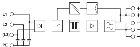
结构框图
