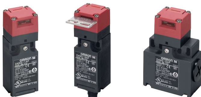
安全门开关
