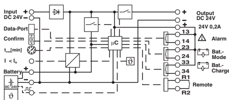
结构框图
