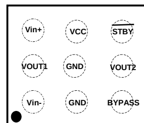
TS4990IST - MiniSO-8
