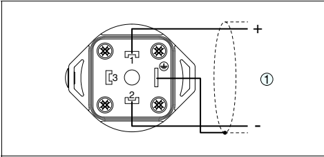
Fig. 29: Versión: Conexión eléctrica "Y", vista en la conexión del lado del equipo
