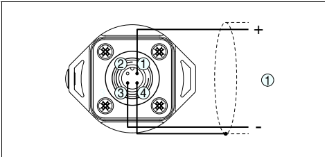
Fig. 30: Versión: Conexión eléctrica "M", vista en la conexión del lado del equipo
