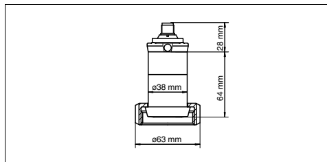
Fig. 23: Version : raccord process „3“, branchement électrique „M“
