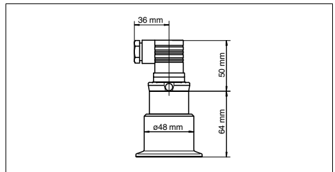
Abb. 8: Ausführung: Prozessanschluss „2“, Elektrischer Anschluss „V“
