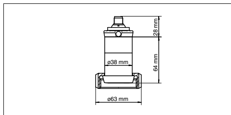
Fig. 31: Versión: Conexión a proceso „3“, Conexión eléctrica „M“
