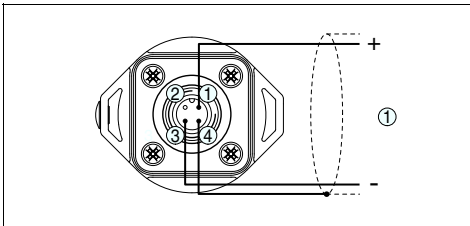
Abb. 6: Ausführung: Elektrischer Anschluss "M", Ansicht auf den geräteseitigen Anschluss
