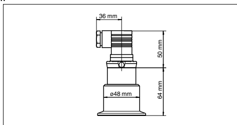
Fig. 24: Version : raccord process „2“, branchement électrique „V“
