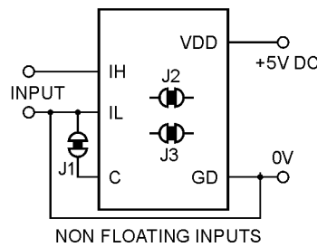
NON FLOATING INPUTS
