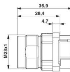
Installation dimensions SF-...P1N8AWK00
