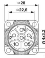
Installation dimensions SF-...P1N8AWK00
