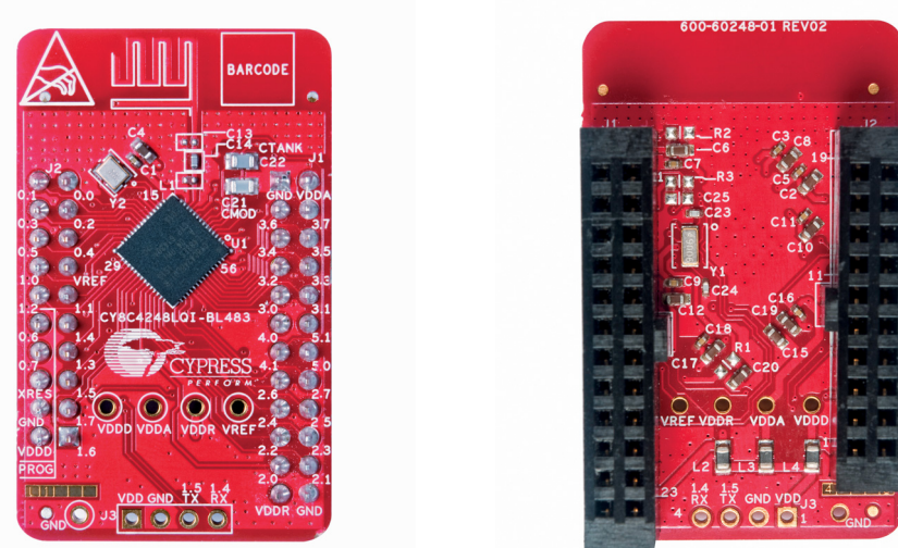
Figure A-5. CY8CKIT-143 PSoC 4 BLE 256KB Module
