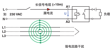
强电回路干扰
