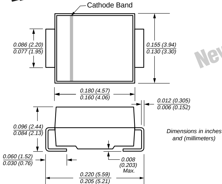
DO-214AA (SMB J-Bend)
