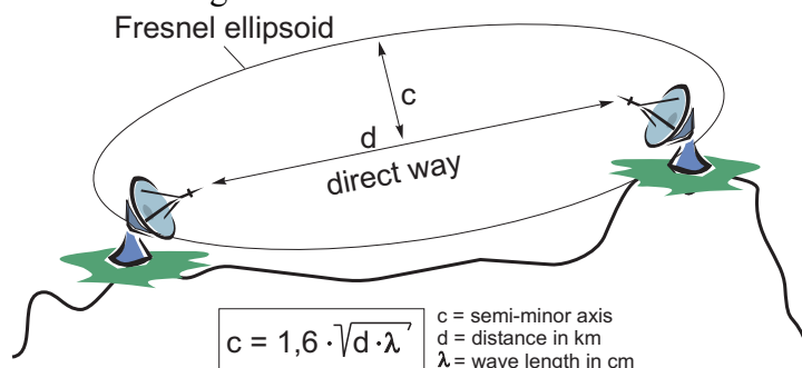
Fig. 2.1.1-6: Fresnel zone
