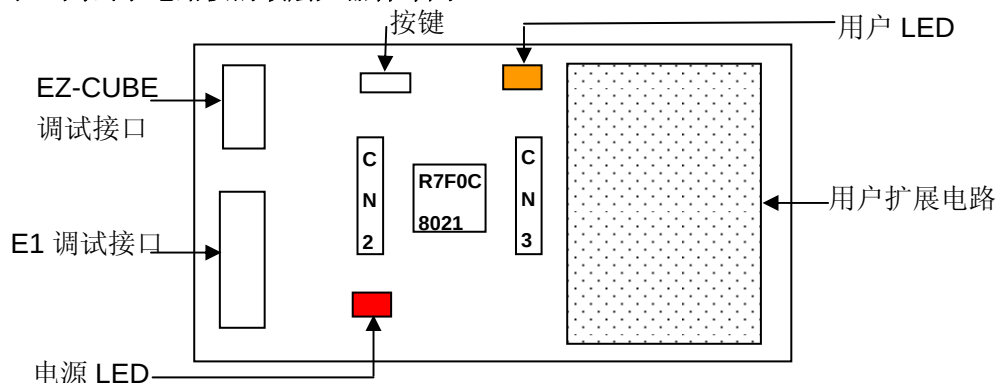
图3-1 电路板布局
