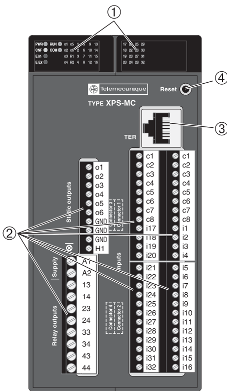
Configuration du couvercle XPS-MC32
