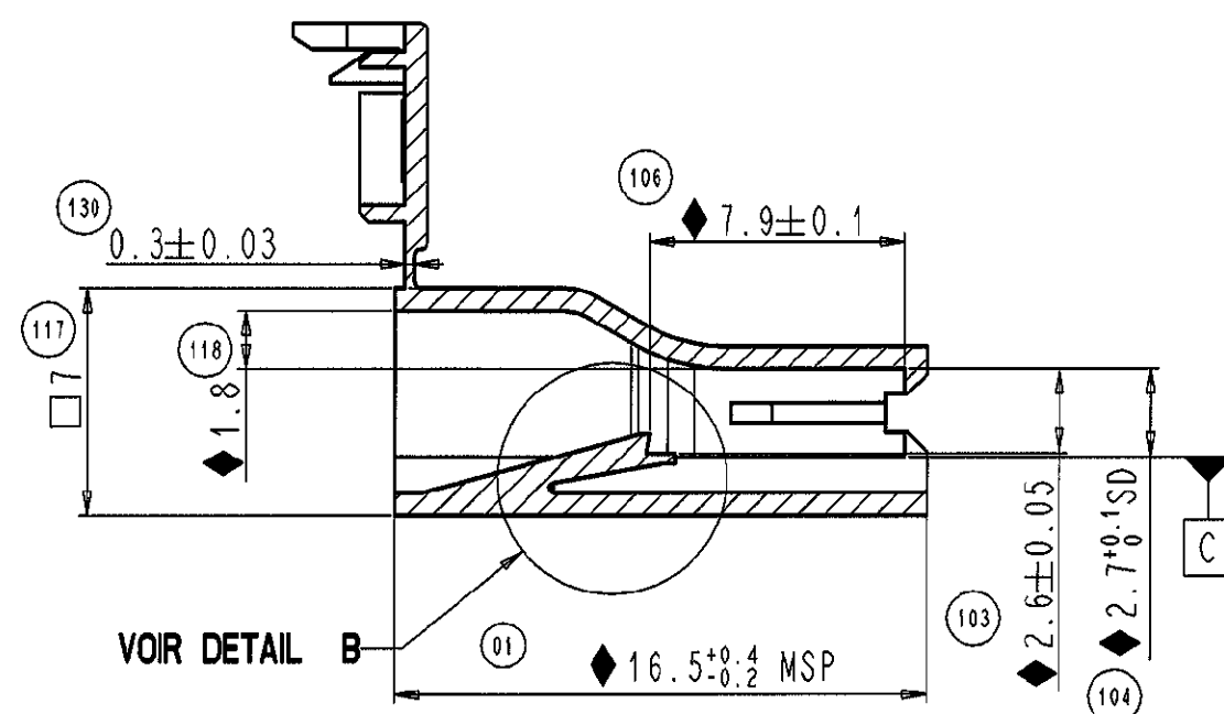
COUPE A-A
