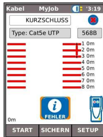
Abb. 26 Kurzschluss nach Pin
