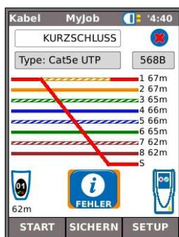
Abb. 31 Überbrückte Kurzschlüsse
