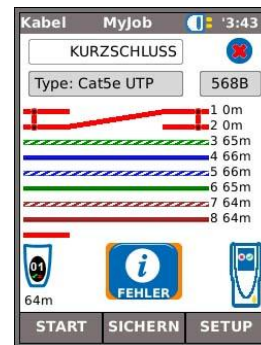
Abb. 28 Kurzschluss nach Pin
