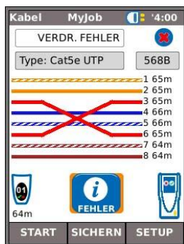
Abb. 29 Gekreuzte Paare
