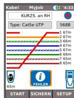
Abb. 32 Remote Kurzschlüsse
