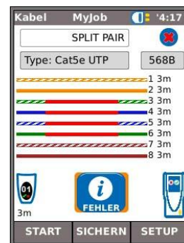
Abb. 30 Split-Paare
