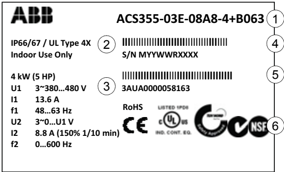
Etiqueta de designación de tipo
