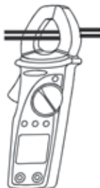
Abb. 6: Verwendung der Zange für Gleichstrommessungen
