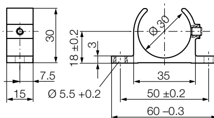
Figura 7-1: Pinza de fijación BTL6-A-MF01-A-50
