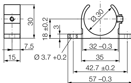
Figura 7-2: Pinza de fijación BTL6-A-MF01-A-43
