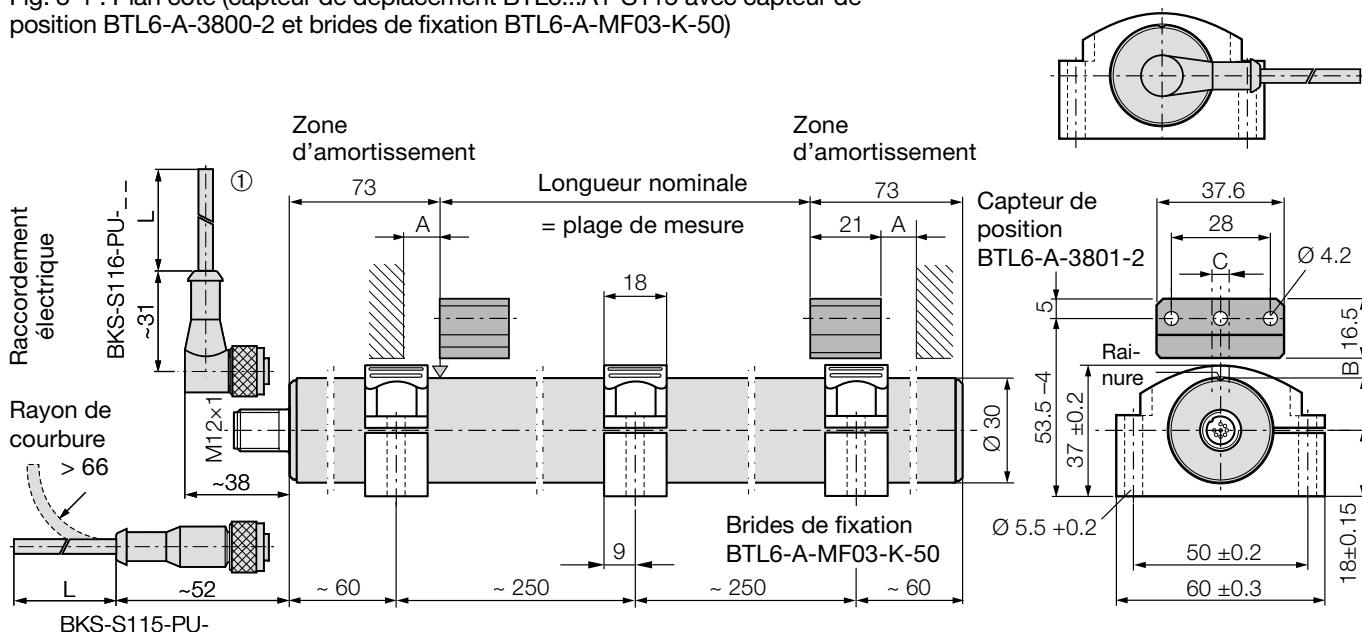
Fig. 3-2 : Plan coté (capteur de déplacement BTL6...A1-S115 avec capteur de position BTL6-A-3801-2 et brides de fixation BTL6-A-MF03-K-50)
