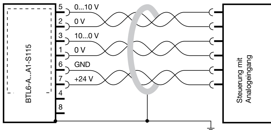
Bild 4-1: Anschlussbeispiel BTL6-A...A1-S115 mit Steuerung
