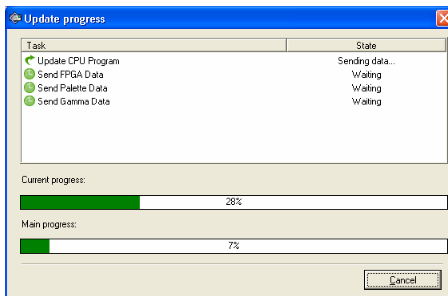
Fig. 5.61 Update Progress
