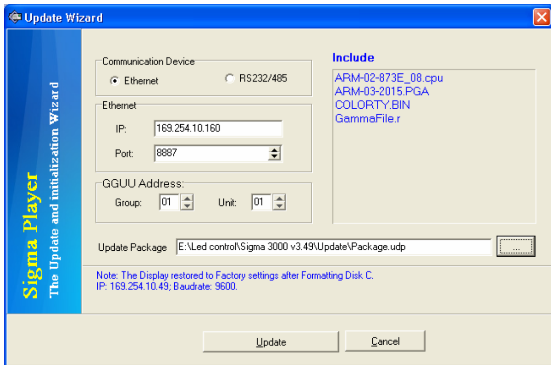
Fig. 5.60 Update Wizard
