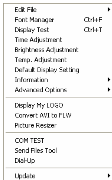
Fig. 5.19 Tool Menu
