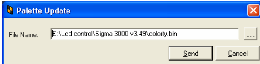
Fig. 5.58 Palette Update
