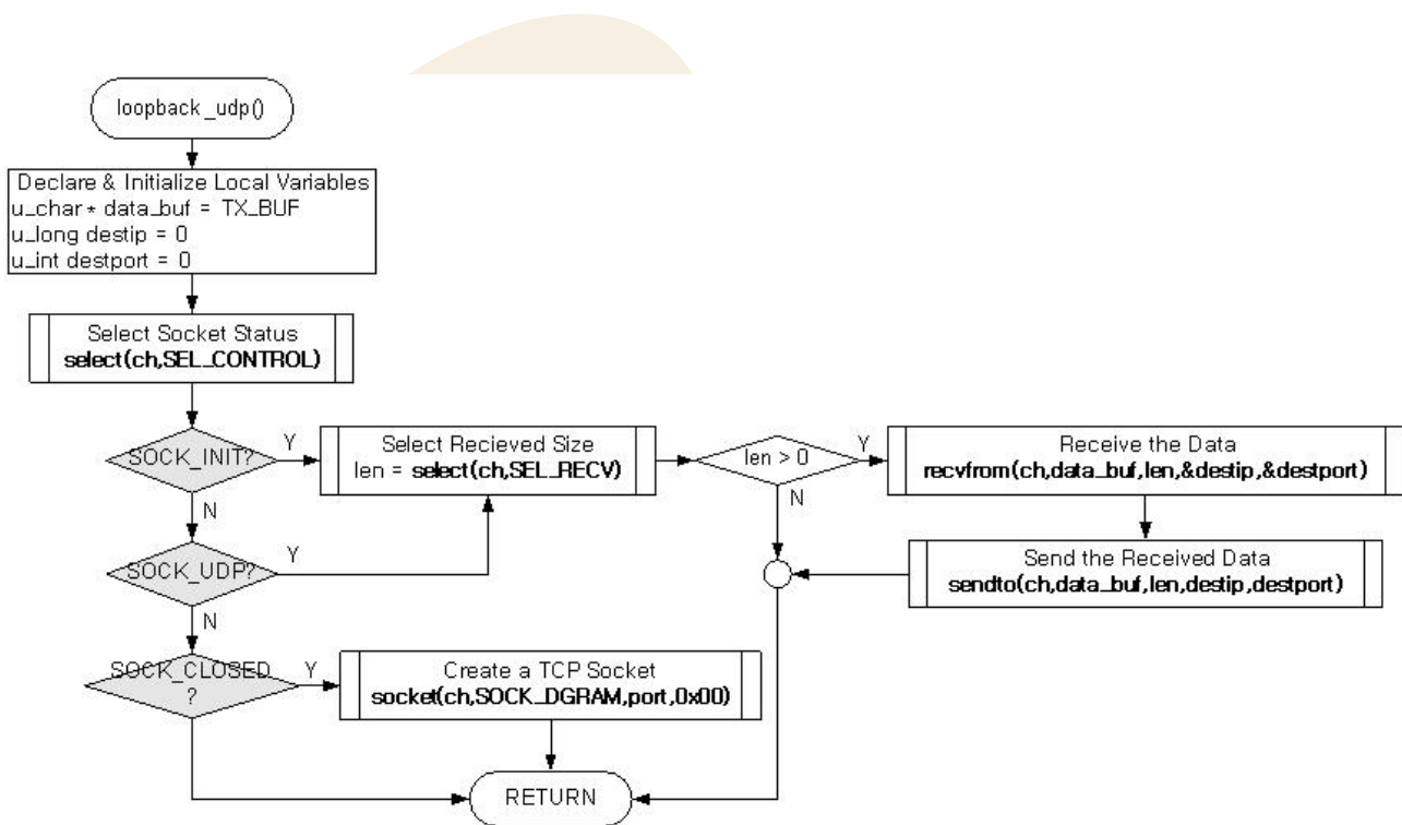
<Fig 3.16: loopback_udp()>
