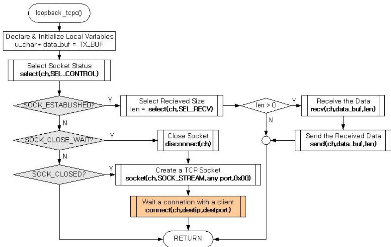
<Fig 3.15: loopback_tcp()>
