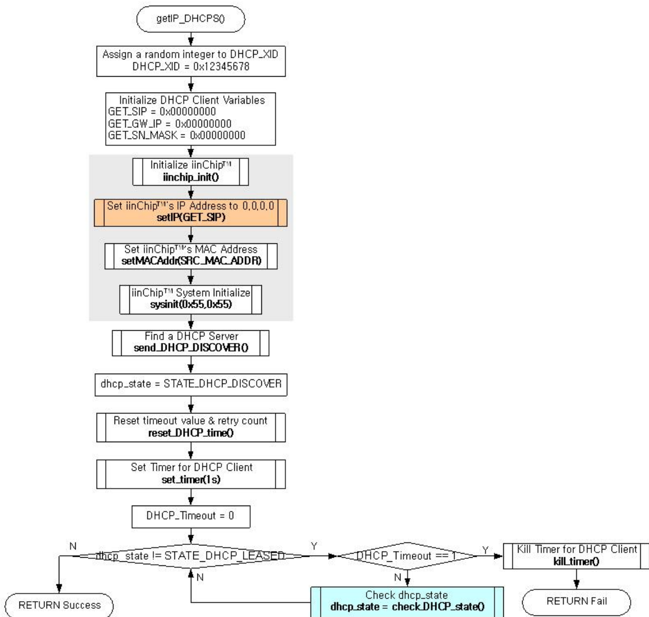
<Fig 3.29: getIP_DHCP()>
