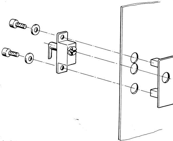
Face avant Plexiglas (coffret compac)
