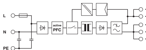
结构框图
