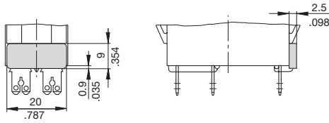
Terminal adapter Y 303 862 01
